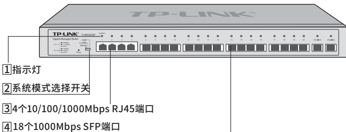
图1-9 TL-SG2422F前面板示意图
